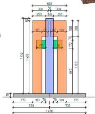
ВИД СПЕРЕД
