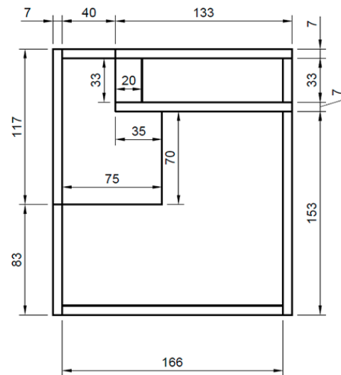
ВИД СВЕРХУ
